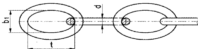
Oblika Art. 20 - ravni člen
